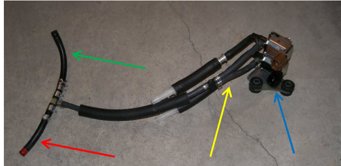
Εικόνα 70: Σωληνάκια ελέγχου waste gate
