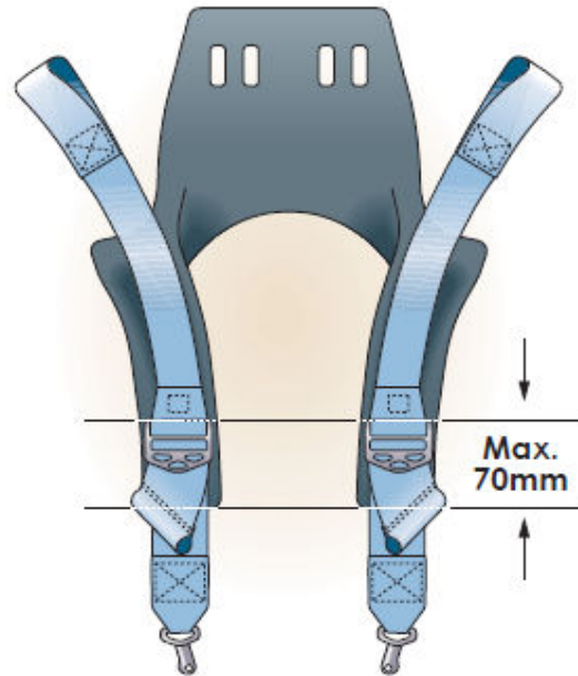
Εικόνα 49: Τοποθέτηση πόρνης σφιξίματος ζώνης ασφαλείας σε σχέση με FHR
