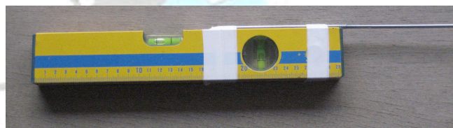
Εικόνα 4: Αλφάδι με βέργα – προέκταση για μέτρηση ύψους ανάρτησης
