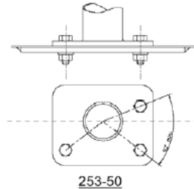
Εικόνα 31: Γωνία βιδών στήριξης κλωβού
