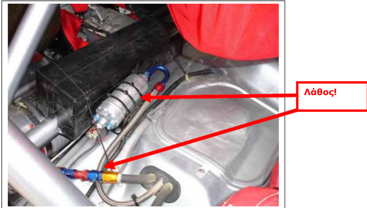
Εικόνα 37: Λανθασμένες σωληνώσεις καυσίμου και αντλία εντός θαλάμου επιβατών
