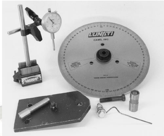
Εικόνα 88: Διάταξη μέτρησης εκκεντροφόρων
