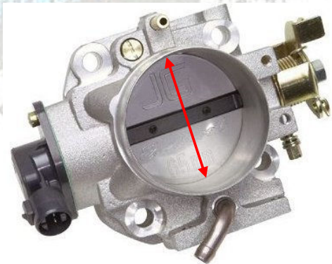
Εικόνα 84: Διάμετρος πεταλούδας εισαγωγής
