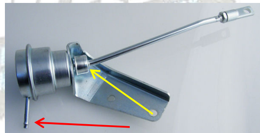
Εικόνα 71: Waste gate
