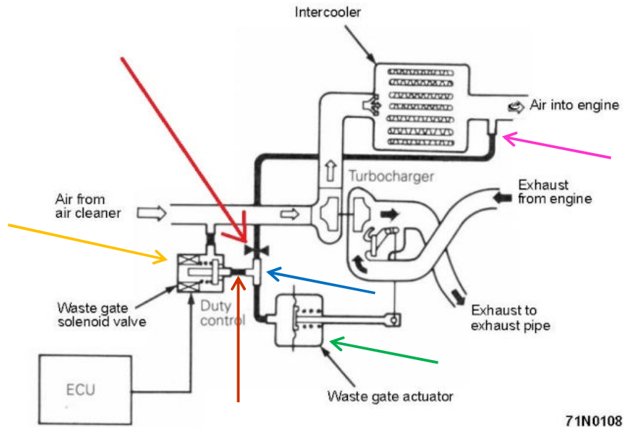
Εικόνα 69: Έλεγχος waste gate
