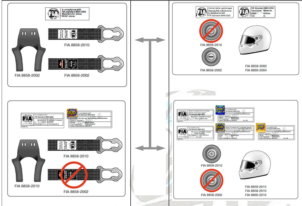
Εικόνα 47: Συμβατότητα προτύπων FHR
