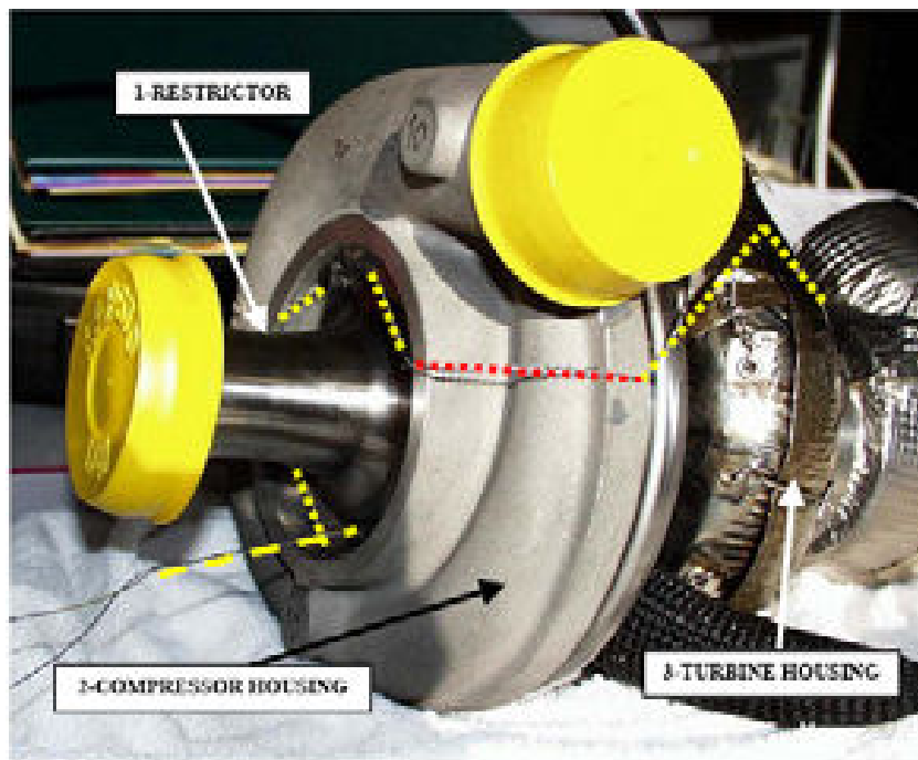
Εικόνα 44: Σφράγιση turbo
