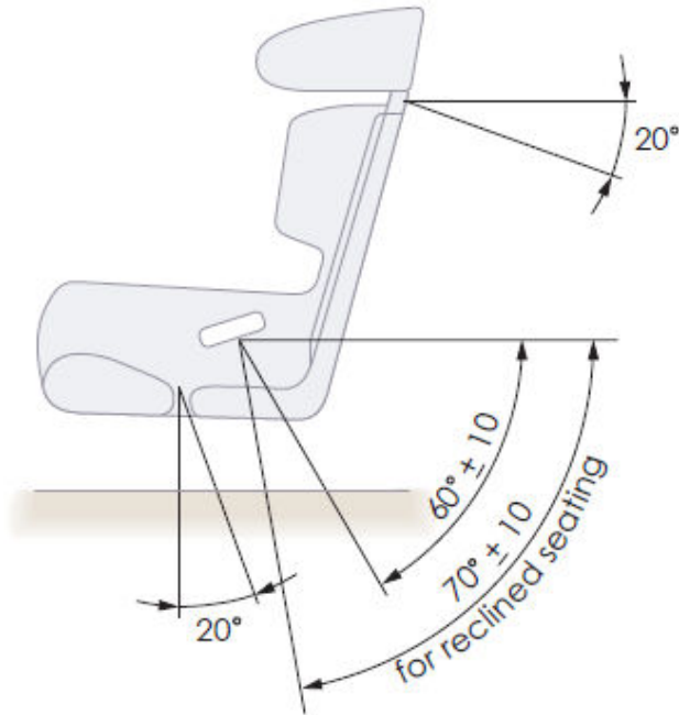
Εικόνα 48: Συνιστώμενες γωνίες ζωνών ασφαλείας για χρήση FHR
