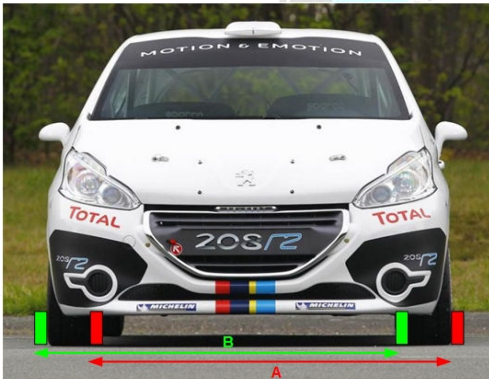
Εικόνα 54: Μέτρηση μετατροχίου
