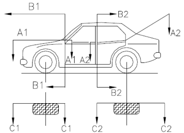
Σχήμα 1: Ορισμός φτερού
