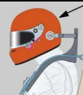
Fig 1 – Etiquette permettant d'identifier les casques équipés dès l'origine des inserts Hans®. Fig 1 – Label for identifying helmets originally equipped with Hans® inserts.
